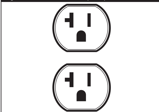
Figura 16 — 120 Volt AC, 20 Amp Receptáculo Doble
