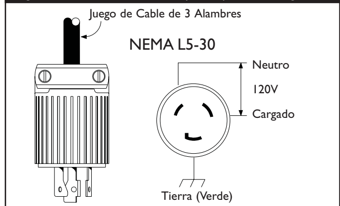
Figura 17 — 120 Volt AC, 30 Amp. Receptáculo de Seguridad
